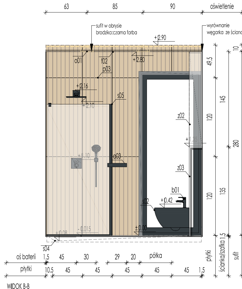
WIDOK B-B
