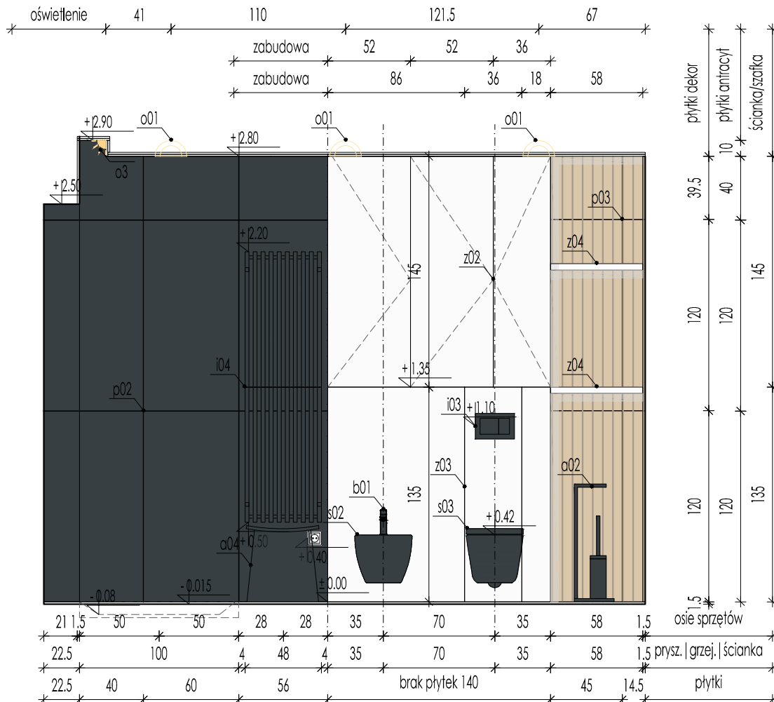
WIDOK C-C
